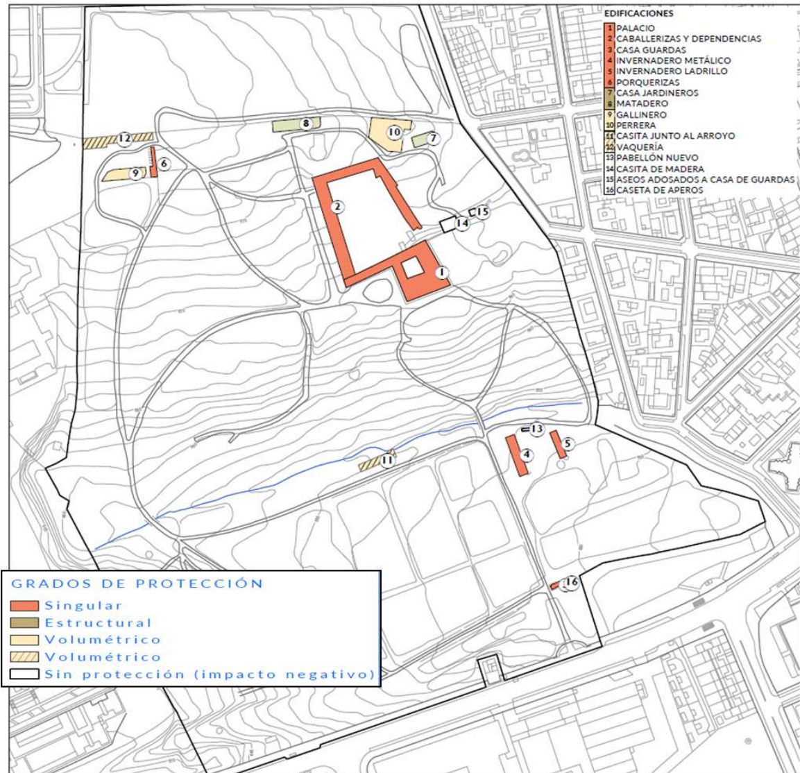
Plano de Catalogación de edificios.
